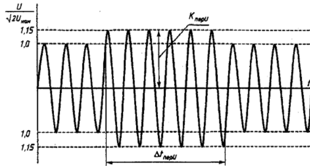
Рисунок Б.4. Временное перенапряжение
